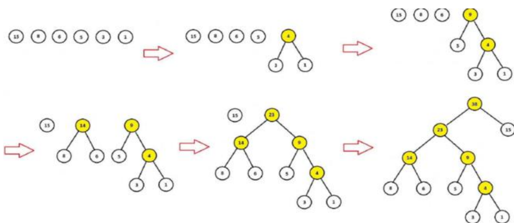
Huffman樹
