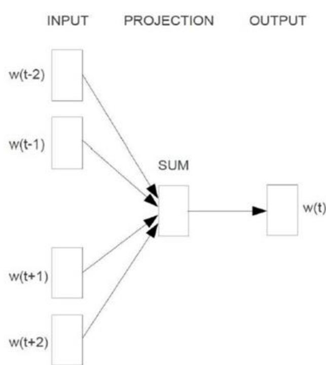
CBOW 模型
